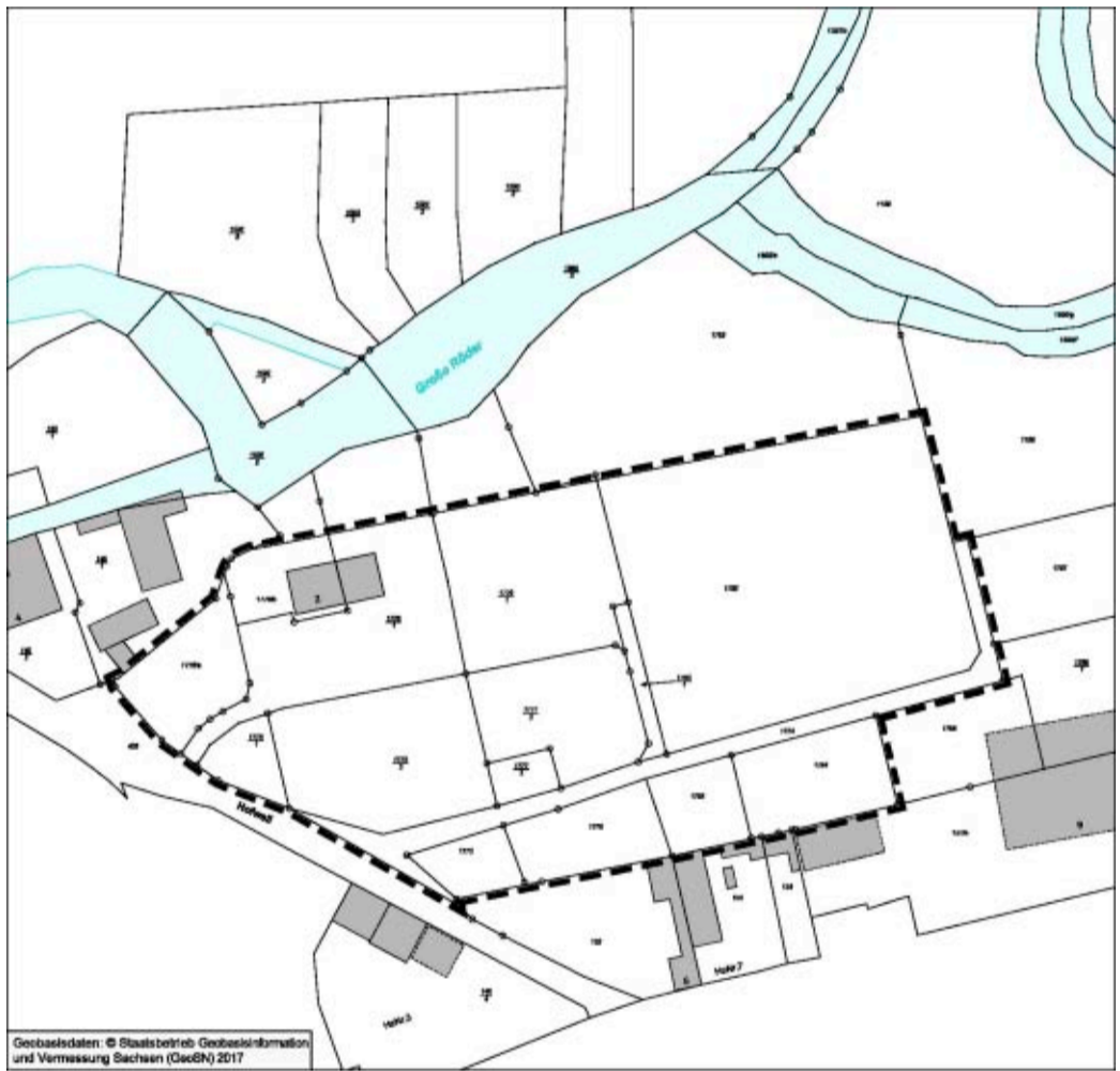
Übersichtsplan - Geltungsbereich Vorhabenbezogener Bebauungsplan „Altenpflegeheim & Wohnen am Hofwall, Radeburg“
